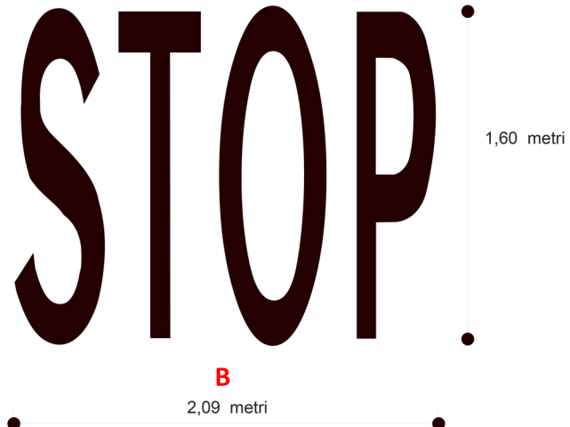
Figura II 441/b Reg. - C.d.S. - Art. 148 ISCRIZIONE DI STOP SU STRADE DI TIPO D-E-F CON V > 50 Km/h
