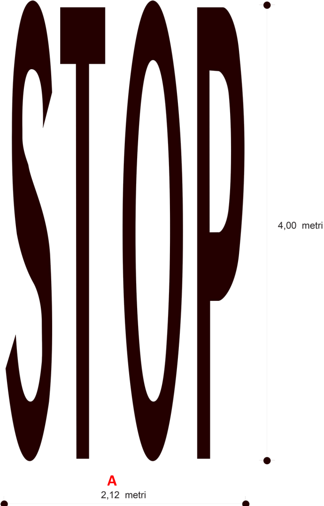
Figura II 441/a Reg. - C.d.S. - Art. 148 ISCRIZIONE DI STOP SU STRADE DI TIPO A-B-C-D CON V > 50 Km/h
